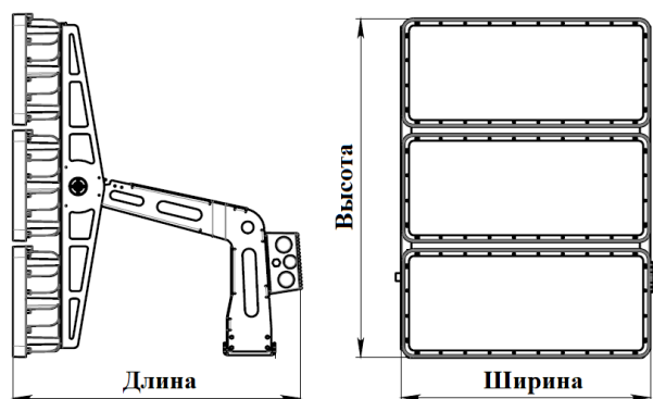
Габаритные размеры
